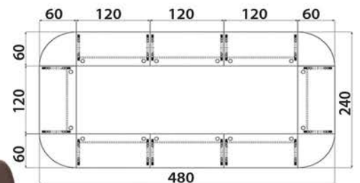
DIMENSION : 480 x 240 x 75 (cm)
